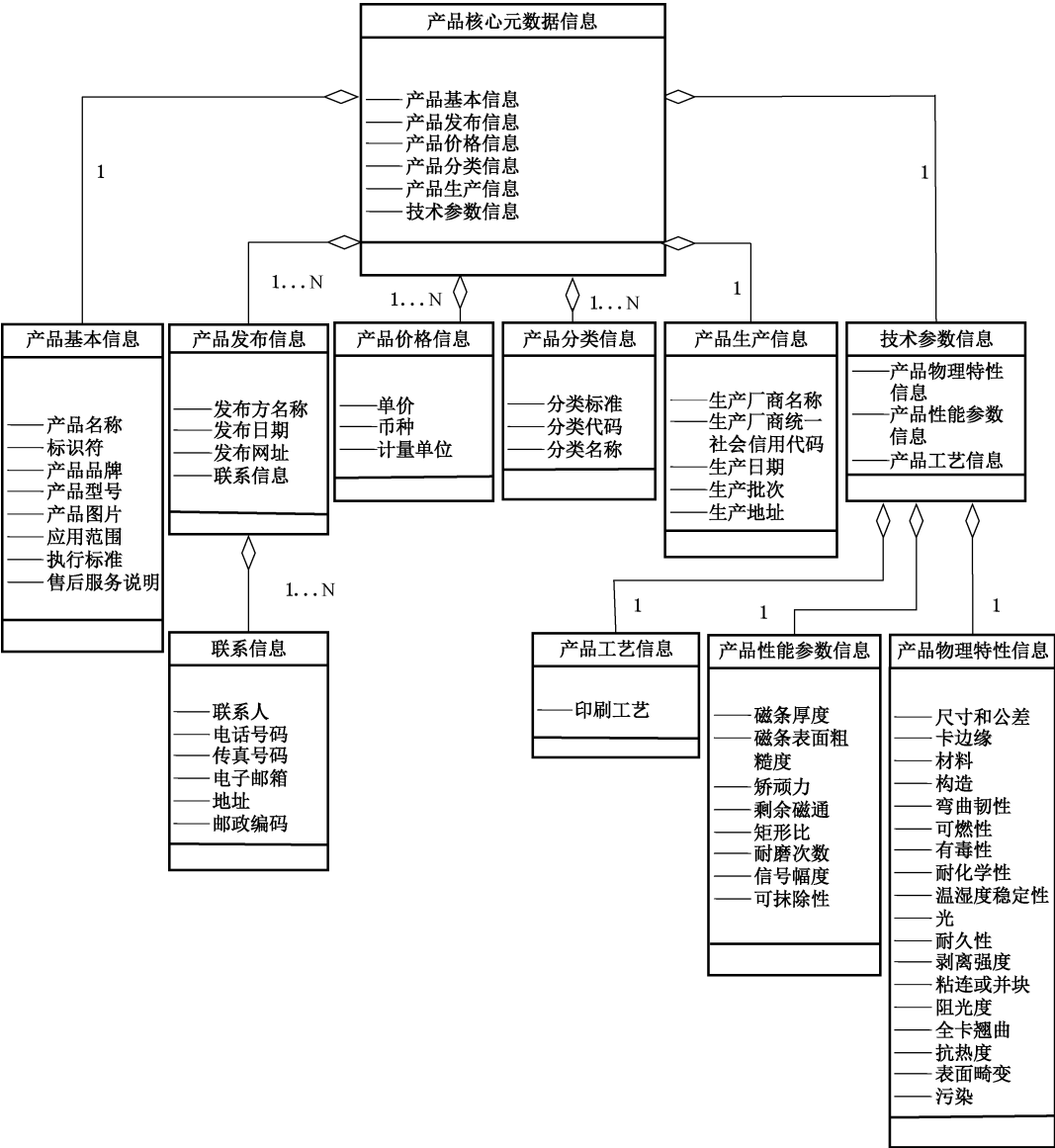
图 1 磁卡产品核心元数据统一建模语言图
